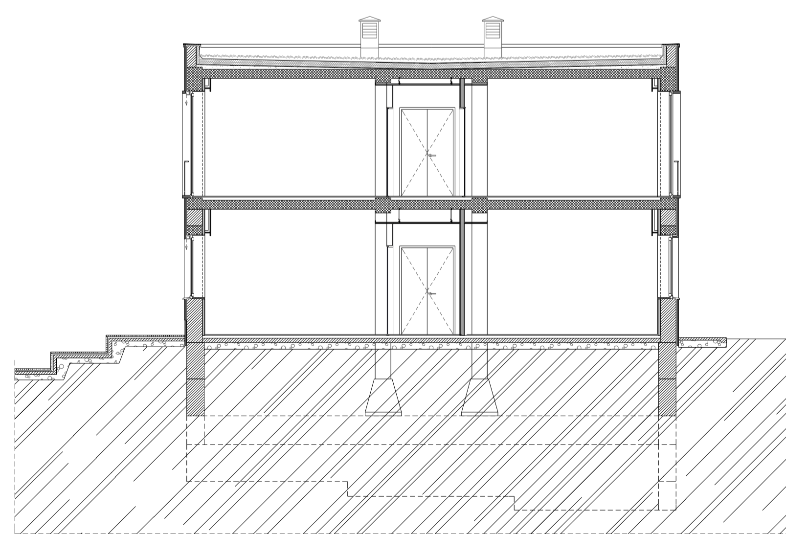
E-E METSZET
