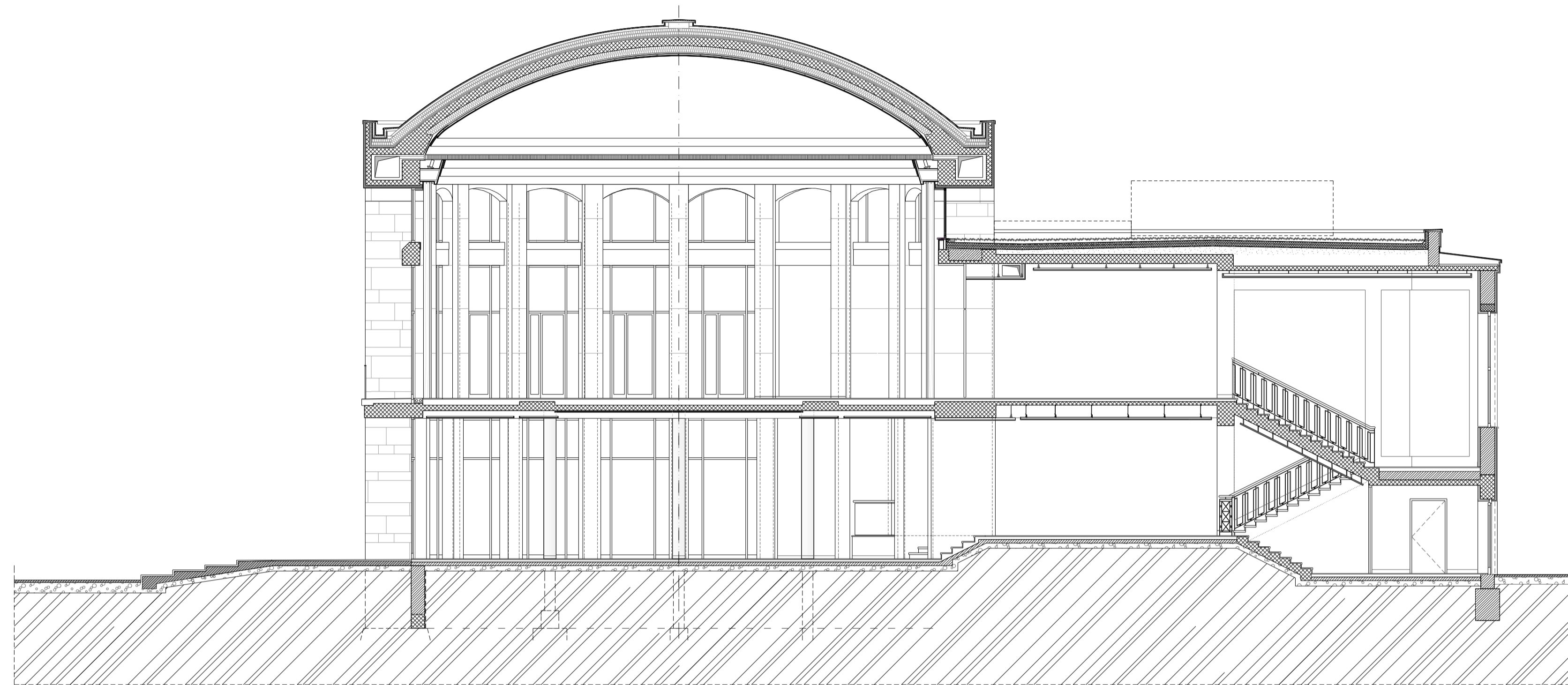
C-C METSZET
