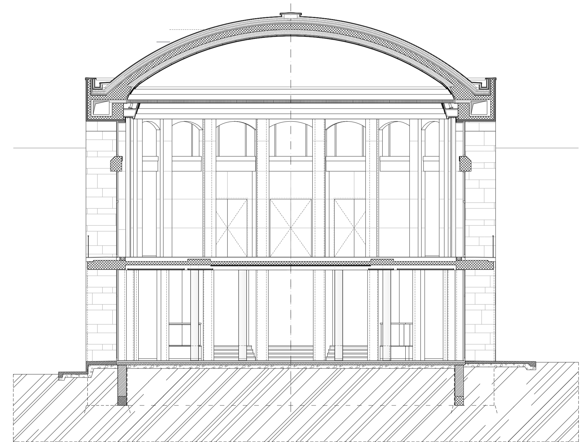
D-D METSZET
