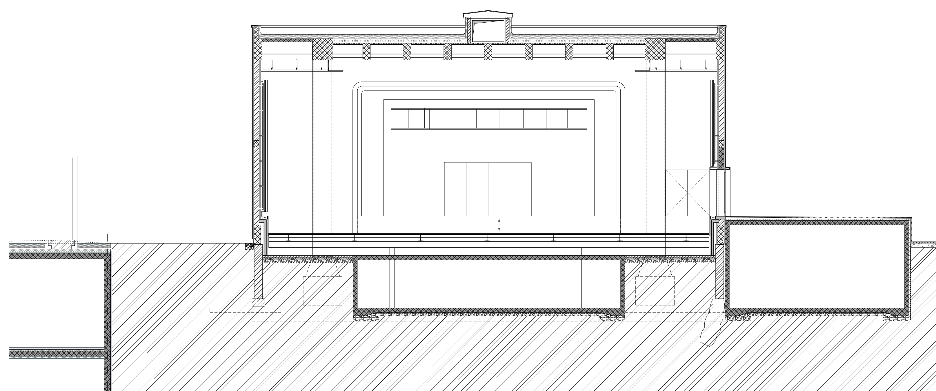
B-B METSZET
