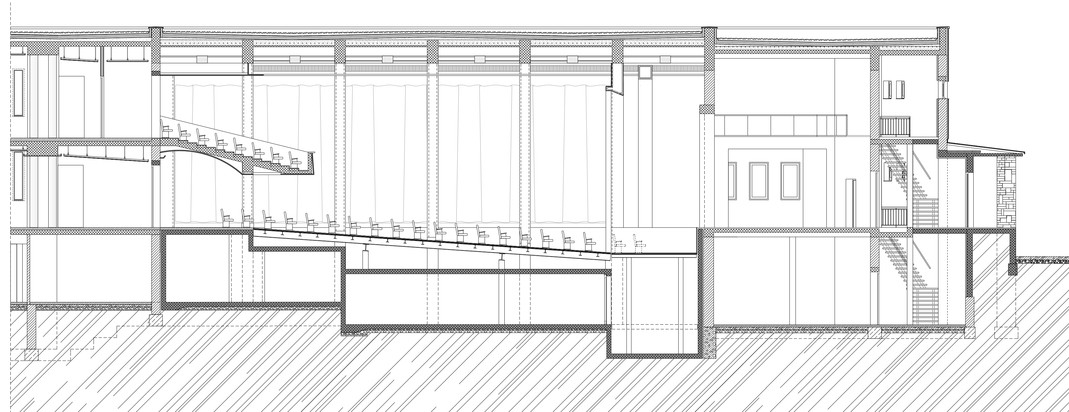
A-A METSZET
